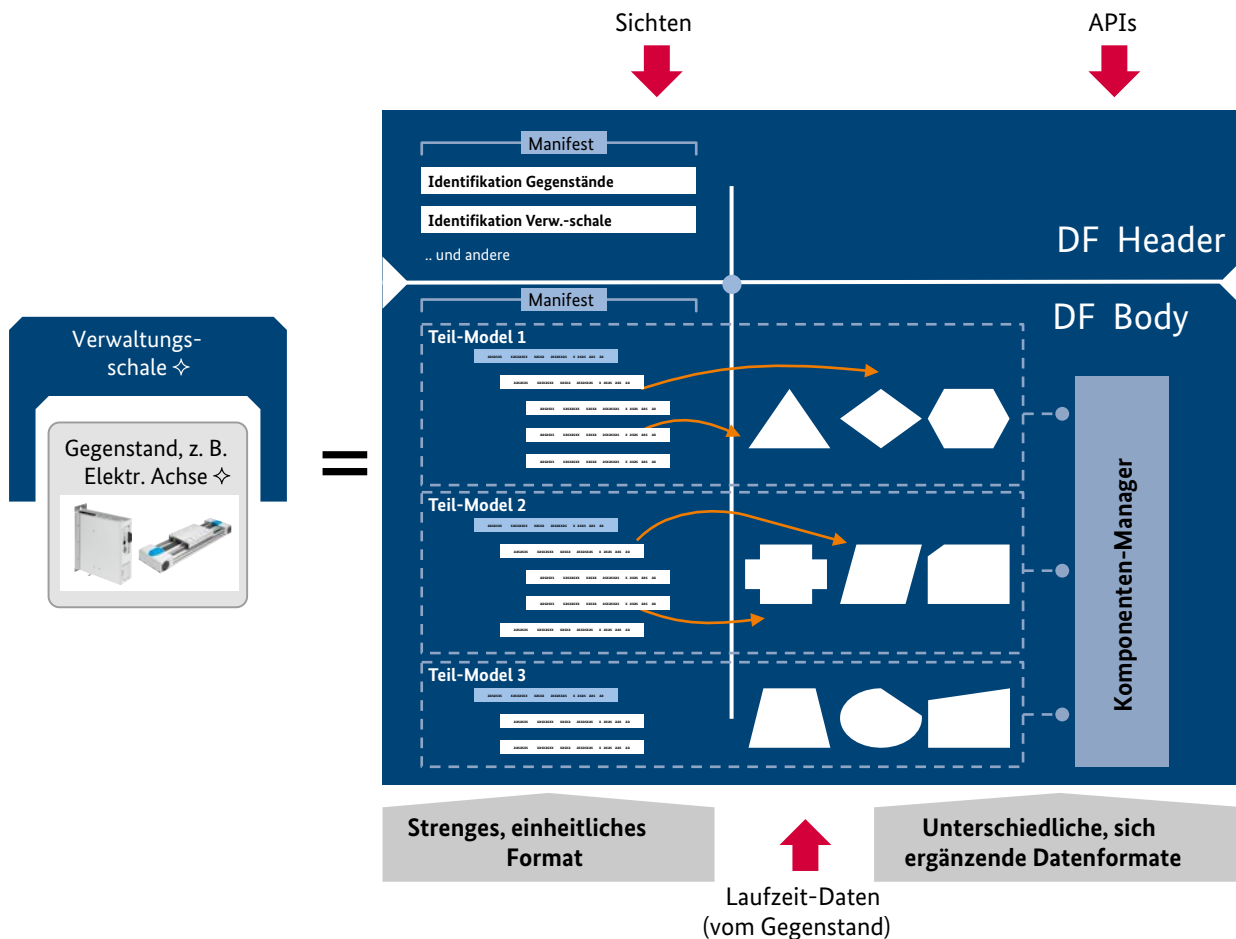
Abbildung 4: Mögliche Header-/Body-Struktur
